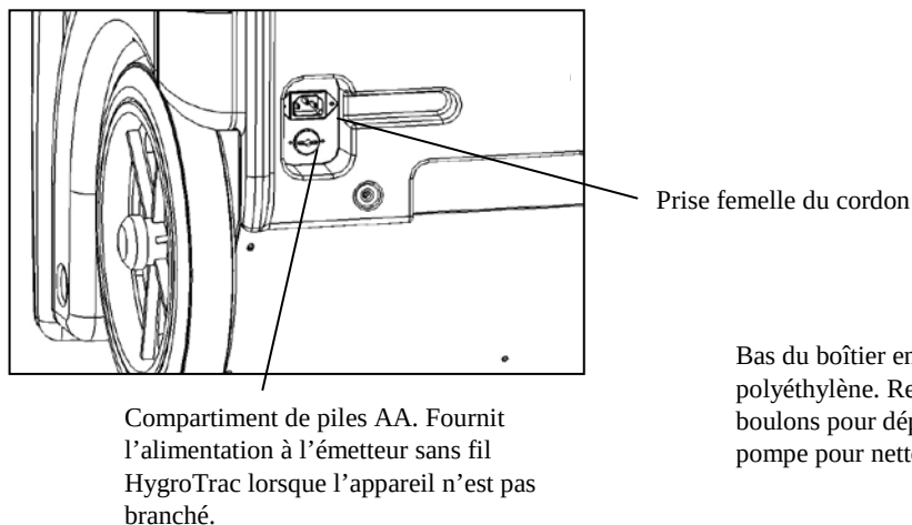
FIG. C : POINTS DE FIXATION DE L'ALIMENTATION ET DE LA POMPE
