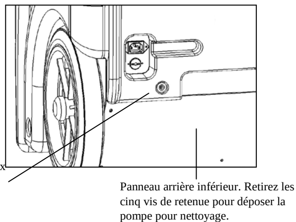
FIG. D : PANNEAU D'ACCÈS DE LA POMPE
