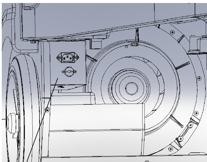
FIG. F : EMBLACEMENT DU BOÎTIER ÉLECTRIQUE
