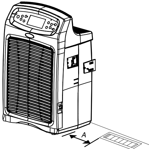
A. Dégagement minimum de 6" (15,2 cm)
